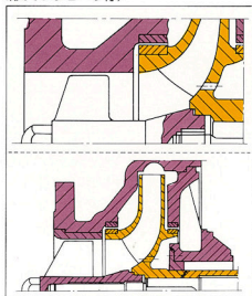
I形(インデューサ付)
