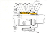
軸封部：バランスメカニカルシール
