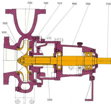
I形(インデューサ付)
