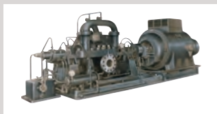
Водяной насос котлами V.M. типа
