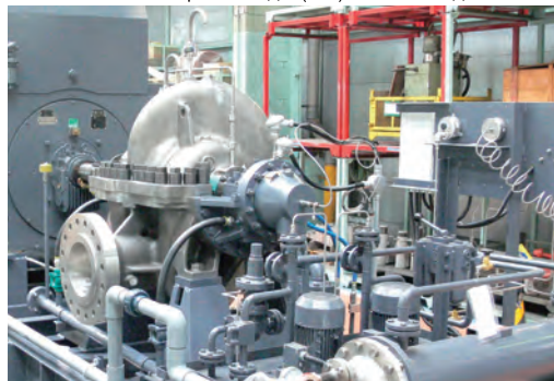
Насос поставки морской воды (RO) с высоким давлением
