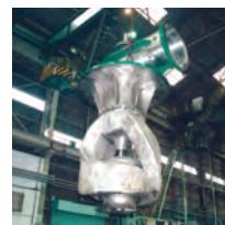
Насос горячего источника для геотермальной электростанции
