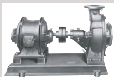
Одноступенчатый, Турбинный насос с одиночным всасыванием
