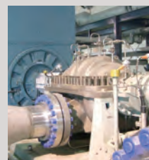
Насос с высоким давлением морской воды для RO опреснения воды в Австралии
