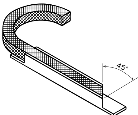
図 4.2-1 グランドパッキンの切断
