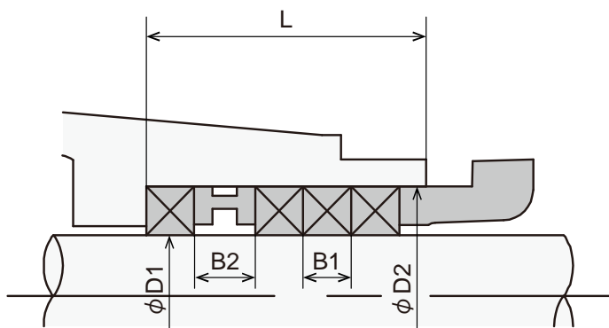
図 4.2-2 軸封部及びグランドパッキンの寸法
