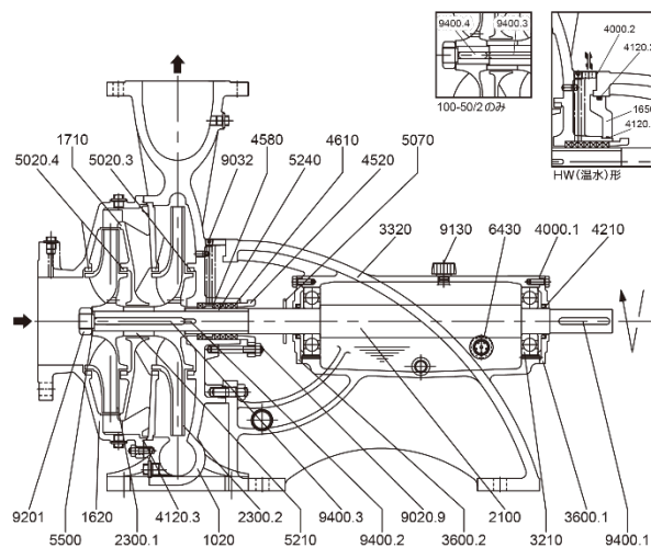
図 1.4-8 2 段スタンド L100、L120
