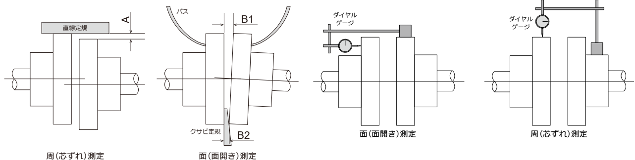
図2.2-1 直線定規、クサビ定規などによる芯出し
