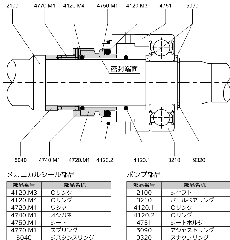
図6.2-1 メカニカルシール構造図
