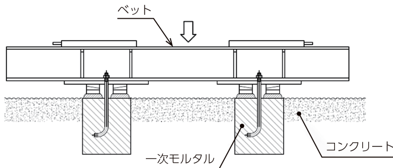
図 2.4-12 ポンプユニットの本据付
