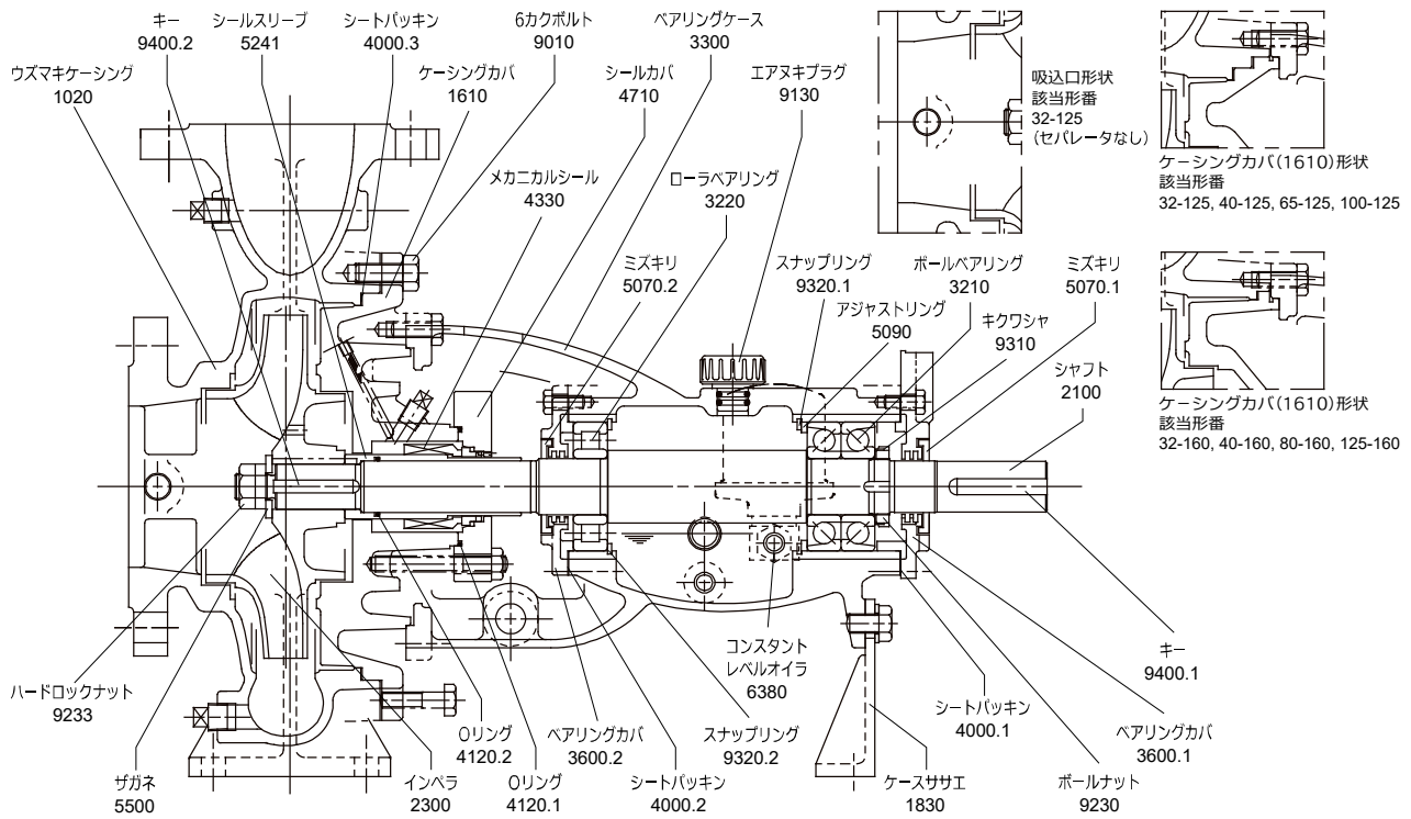
図 1.4-2 グランドパッキン式、グリス潤滑型
