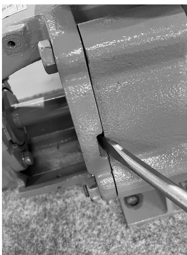
写真 5.2-1 ベアリングケース取り外し
