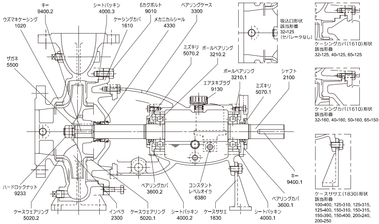
図 1.4-2 CA型メカニカルシール式、オイル潤滑型 (コンスタントレベルオイル式)
