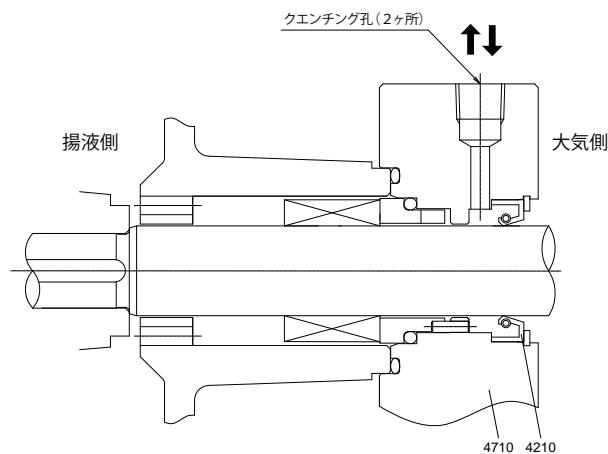
図 6.2-9 クエンチ構造(オイルシール式)
