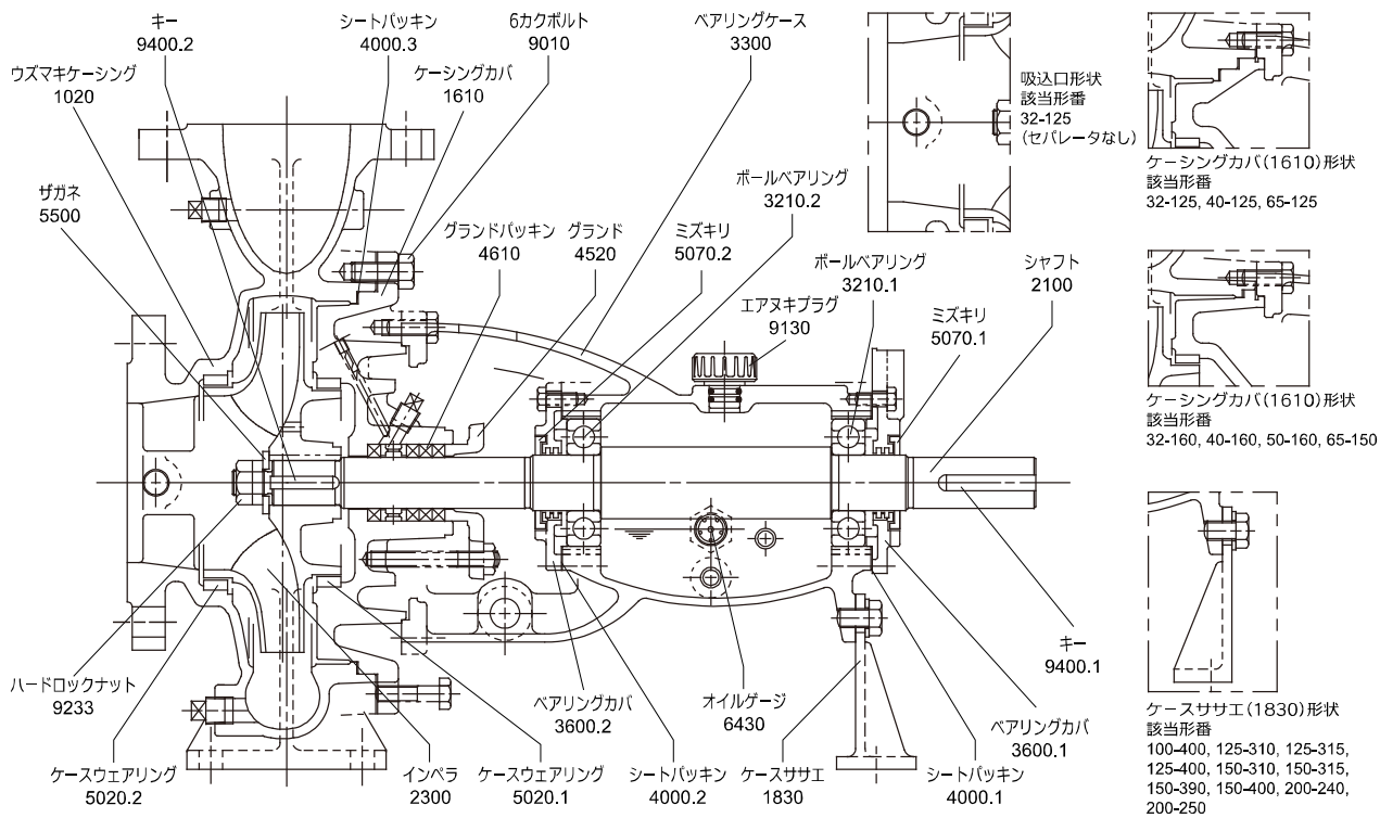
図 1.4-3 グランドパッキン式、オイル潤滑型 (丸型オイルゲージ式)
