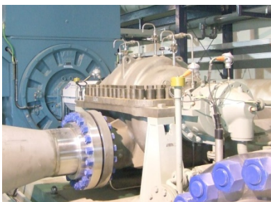
オーストラリア向け高圧海水供給ポンプ
