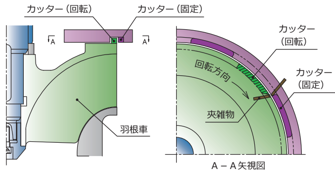
<羽根車 (カッター部) の構造>
