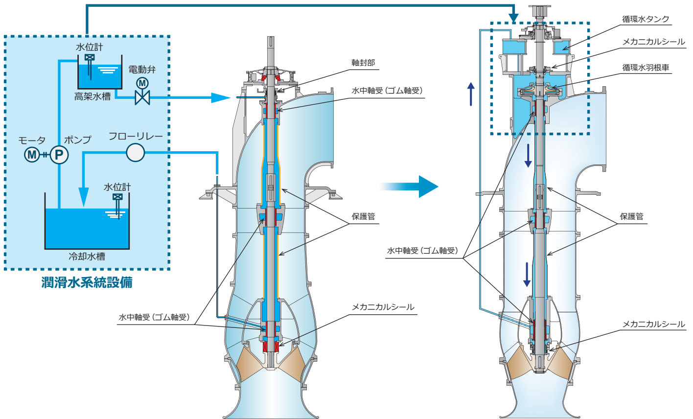
外部注水型立軸ポンプ (従来型)
